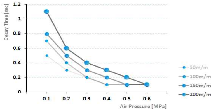
● 본 DATA는 실제 측정값입니다.(±1000V to ±100V / 27°C, 35%)
